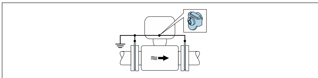
14 Выравнивание потенциалов с помощью заземляющей клеммы и заземляющих дисков
