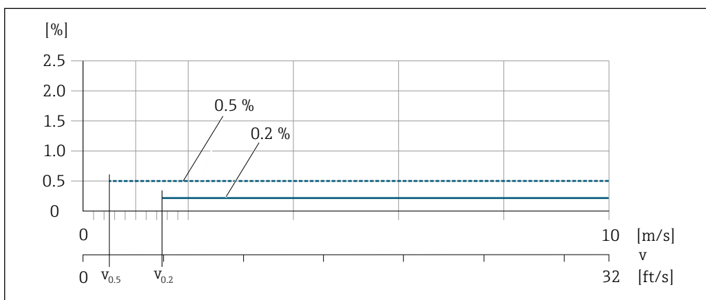
41 Линейная погрешность во всем диапазоне в % ИЗМ
