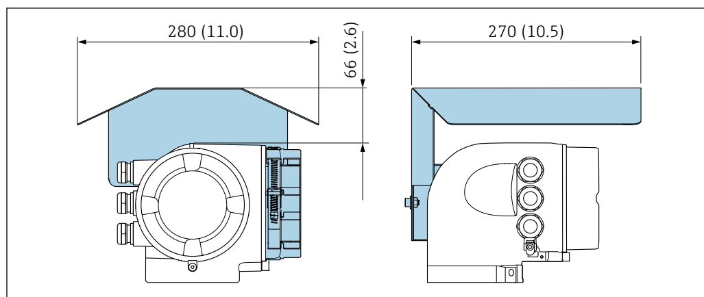
6 Защитный козырек от атмосферных явлений для Proline 500
