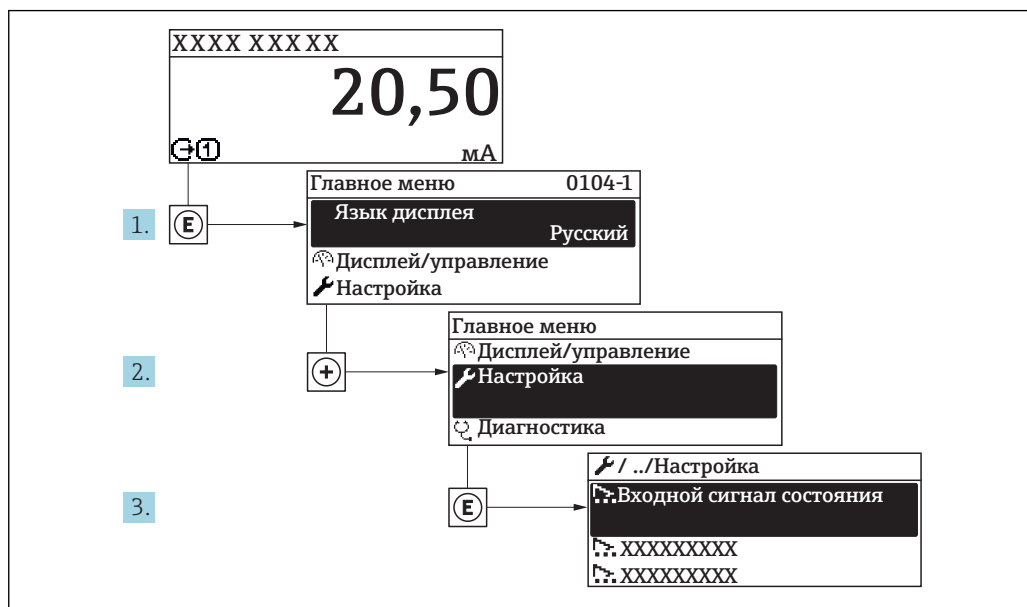
33 Пример индикации на локальном дисплее
